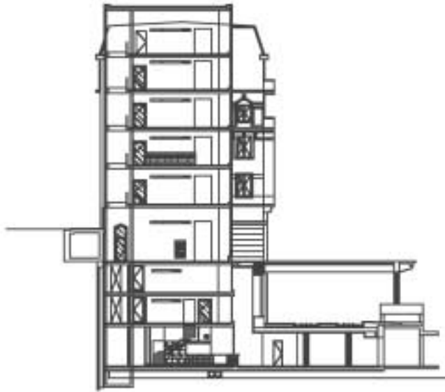
Coupe longitudinale
